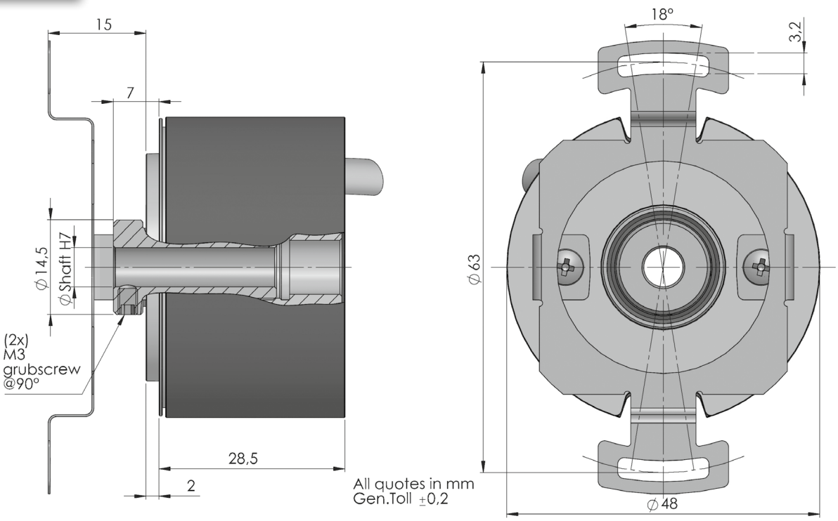
Flansch 3 / Flange 3
