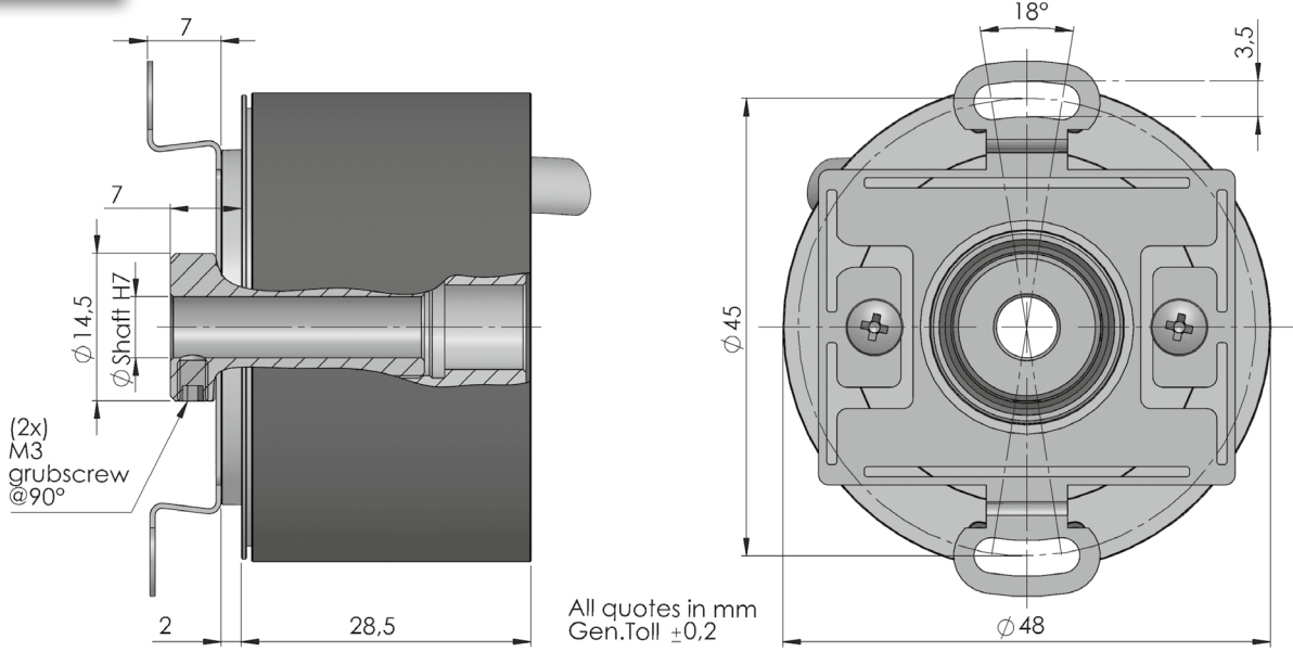
Flansch 2 / Flange 2
