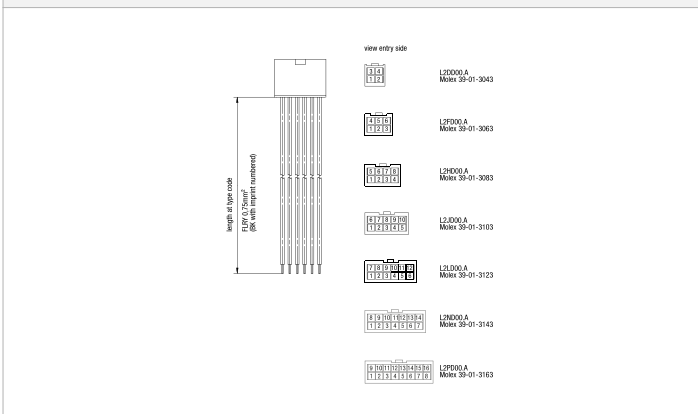
IMAGE 1/2: ANSICHT EINSTECKSEITE, VIEW ENTRY SIDE, VUE FACE D'INSERTION
