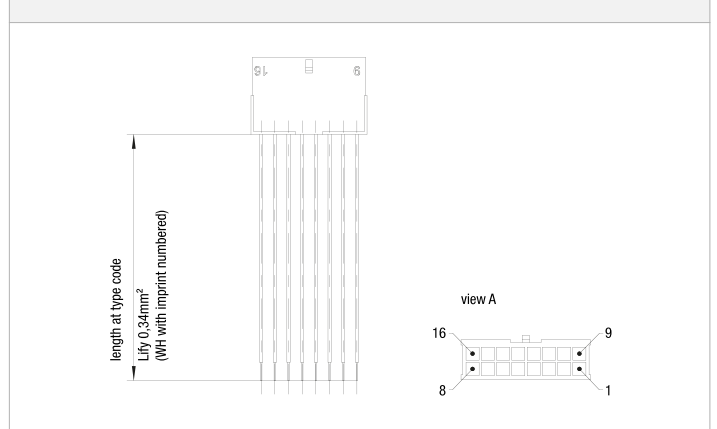
IMAGE 2/2: DETAILANSICHT
